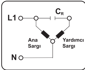
Devre Bağlantısı
