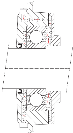
Tahrik Tarafı
