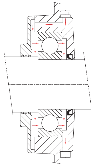
Fan Tarafı
